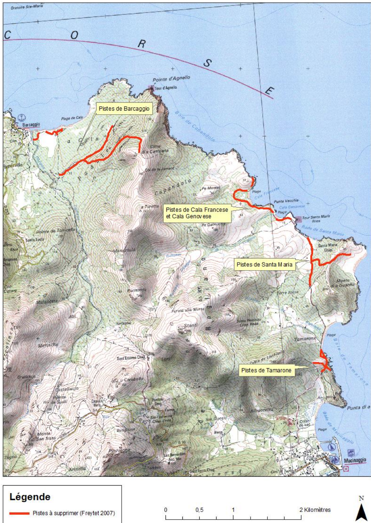
Figure 10. Localisation des pistes à supprimer (Freytet, 2007)
