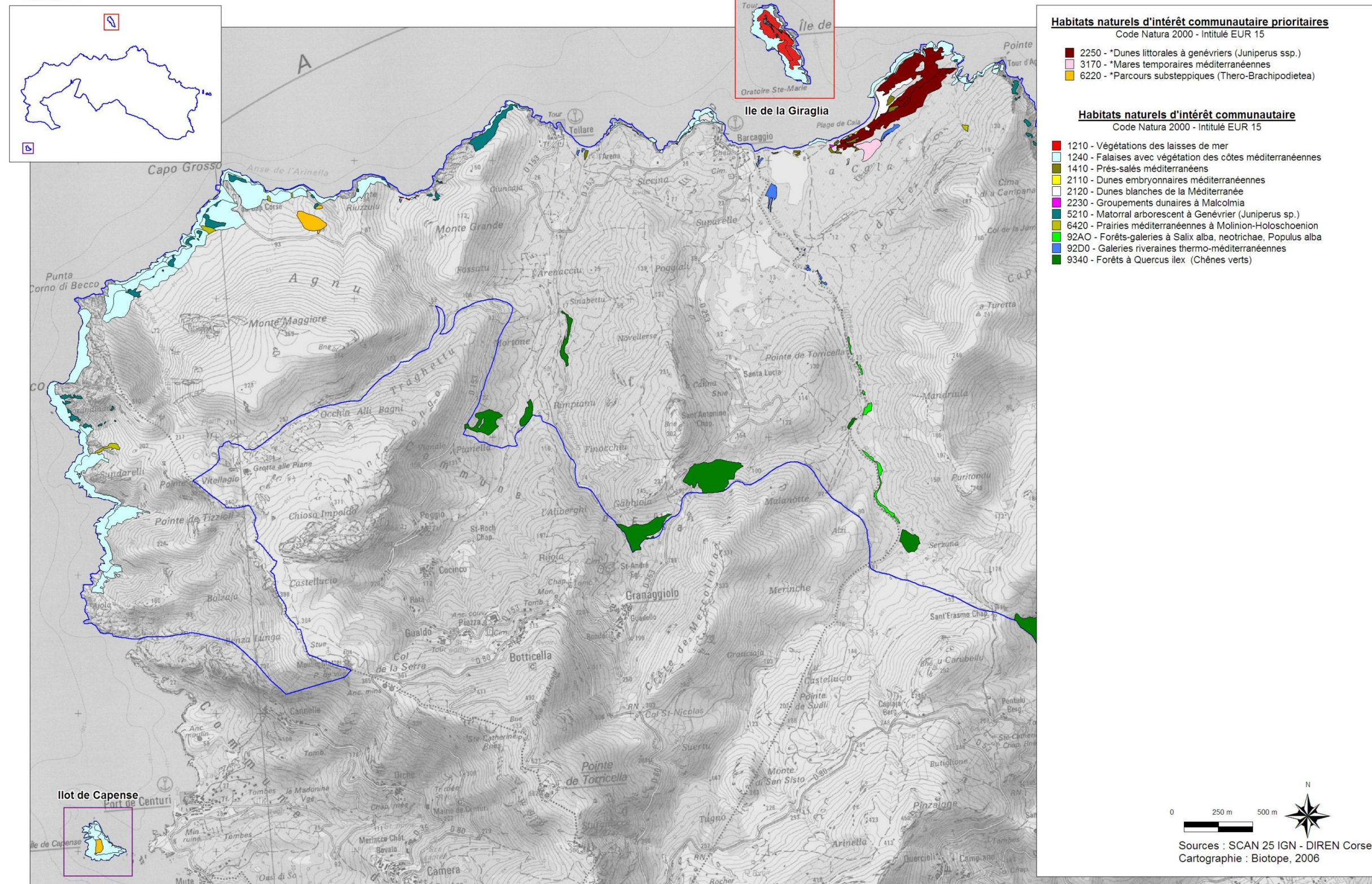
Figure 8. Cartographie des habitats naturels d'intérêt communautaire et prioritaires (partie ouest du site) 3
