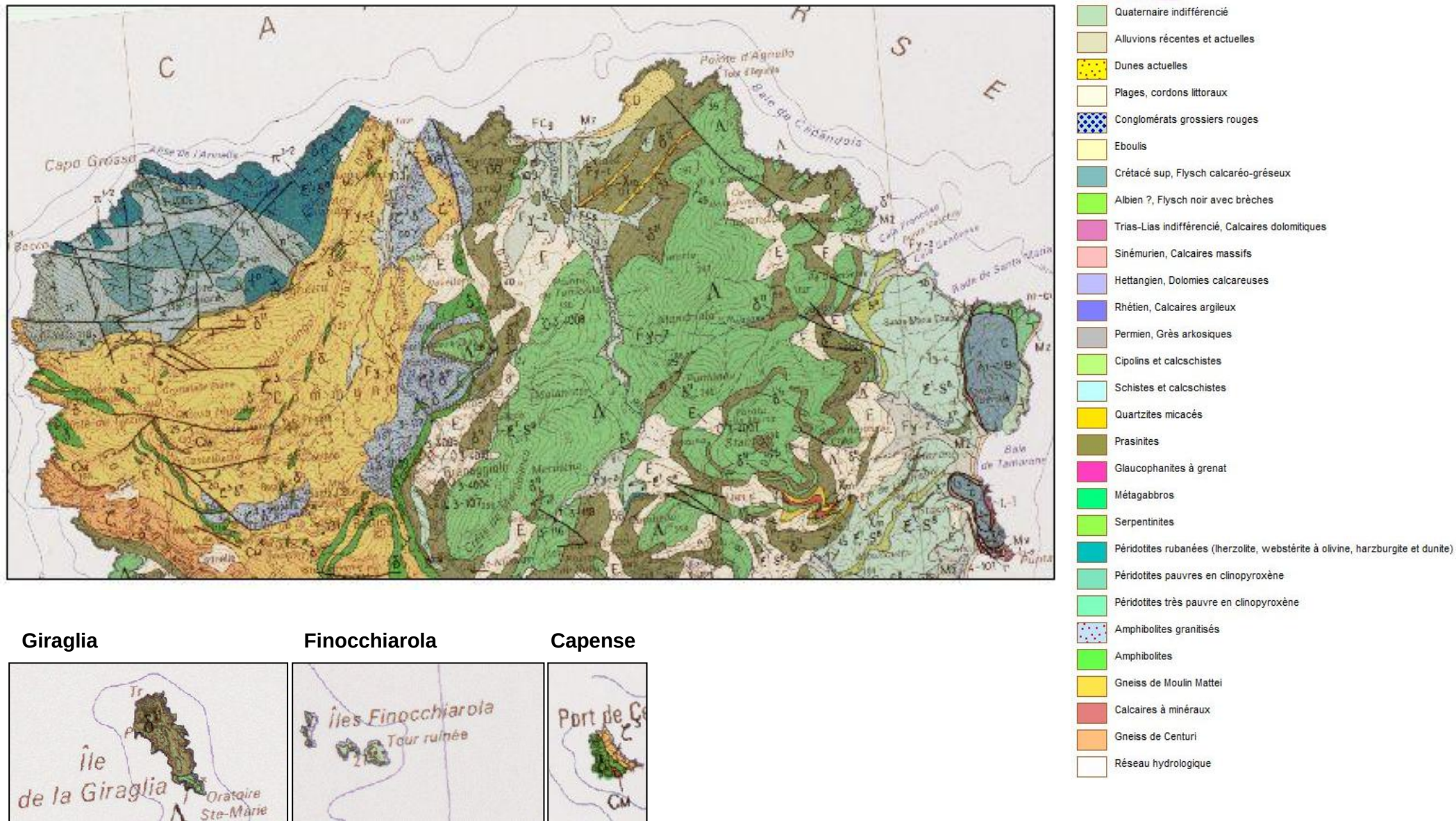
Figure 3. Carte géologique de la Pointe du Cap Corse [Carte géologique imprimée 1/50 000 (BRGM), Topographie France Métropolitaine, Corse et DOM-COM (GEOSIGNAL)]
