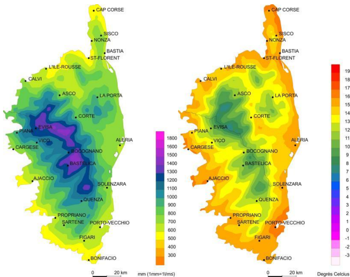
Précipitations annuelles moyennes 1961-1990
