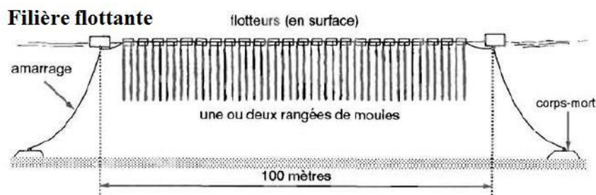
Figure 71 : Principe de la culture de moules sur filière (source IFREMER)
